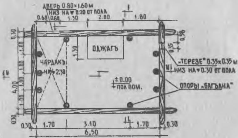
Рис. 15. Старинное карачаевское жилище. План «Уллу-ю».
