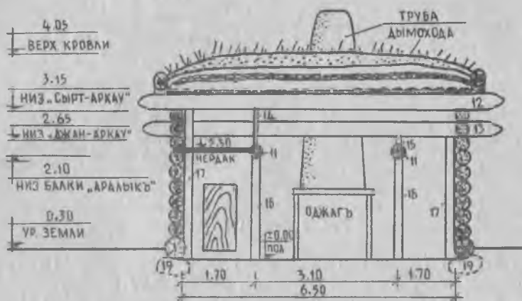
Рис. 17. Продольный разрез II—II. М—1 : 50.
