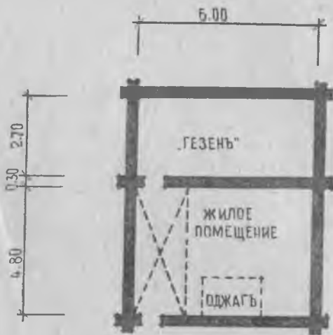
Рис. 28. Очажное помещение с кладовой «гёзен» арбаз Дудова, аул Хурзук. М—1:100.
