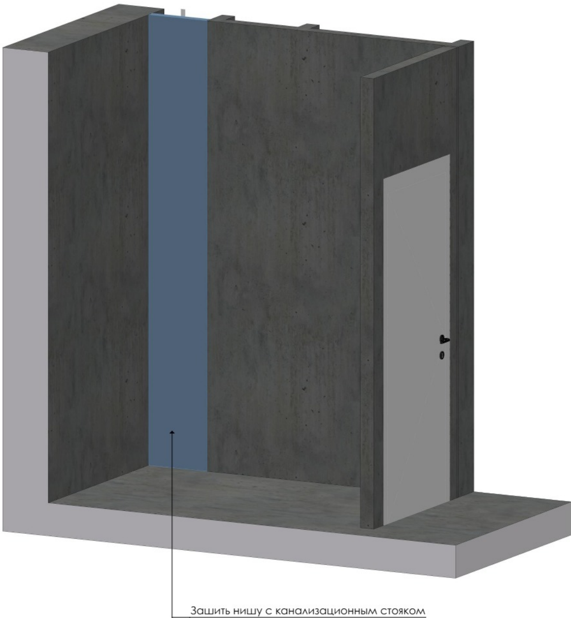
Монтаж ВГКЛ конструкции в постирочной
