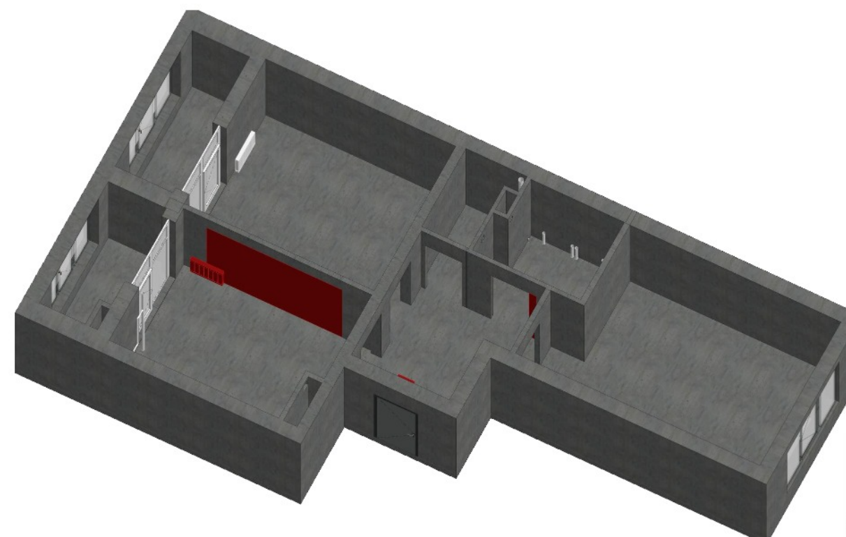
Общий 3D вид плана демонтажа
