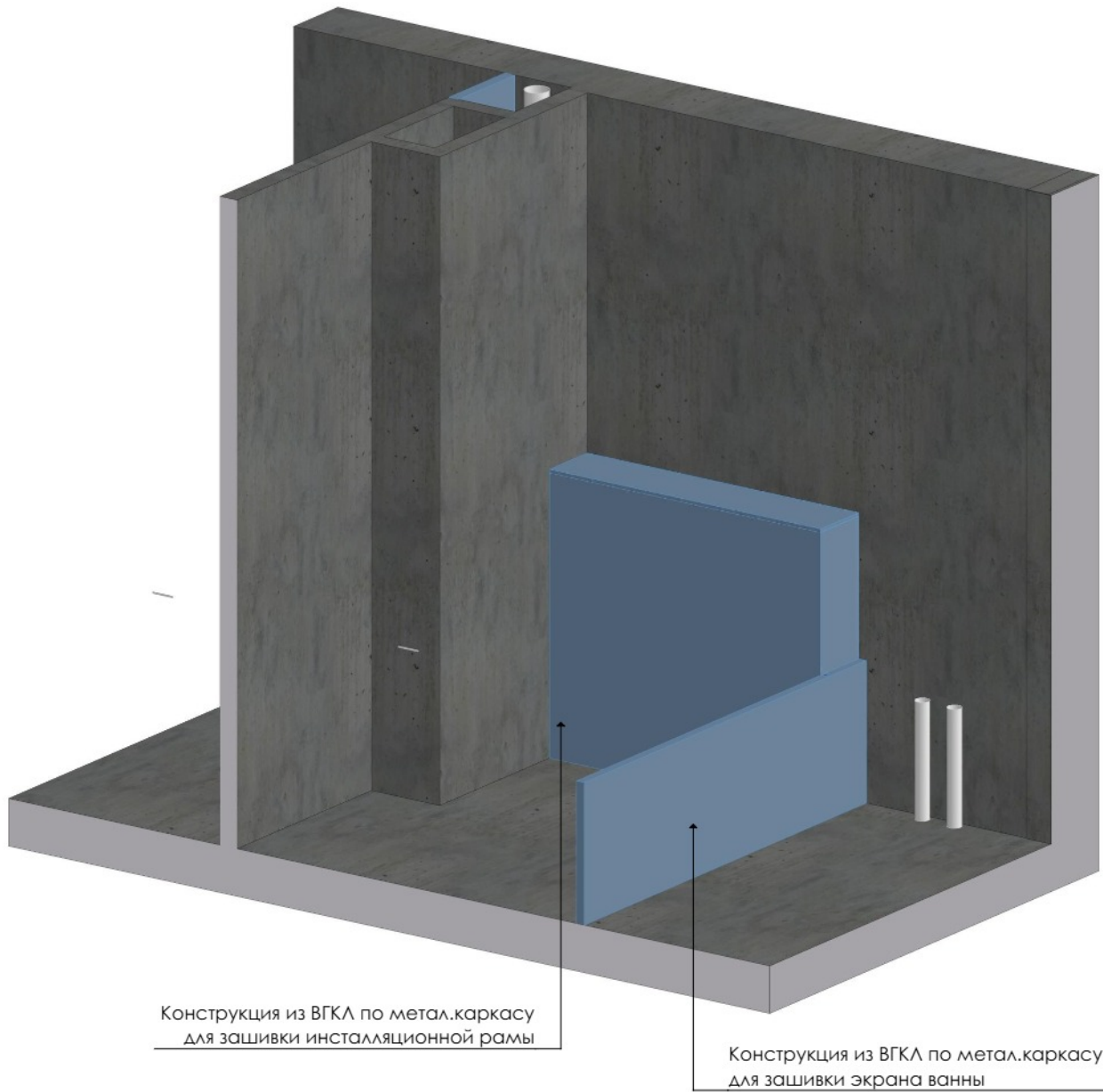
Монтаж ВГКЛ конструкции в ванне
