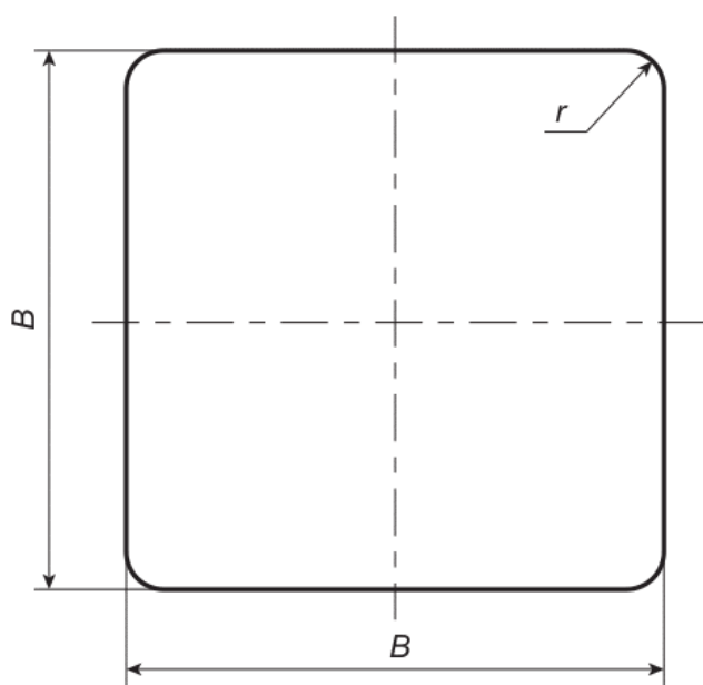
Рисунок Д.5 - Размеры квадратных знаков
