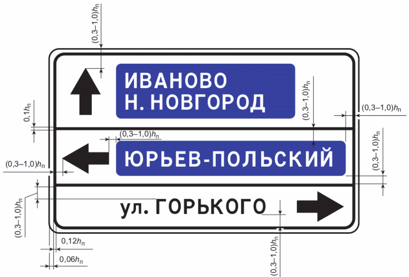
Рисунок Г.4 - Пример компоновки знака индивидуального проектирования 6.10.1
