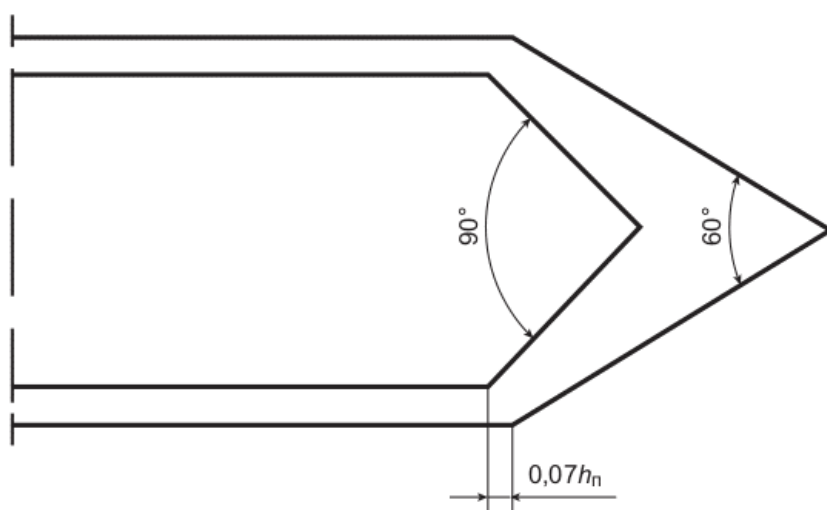
Рисунок Г.2 - Конфигурация оголовка знака индивидуального проектирования 6.10.2
