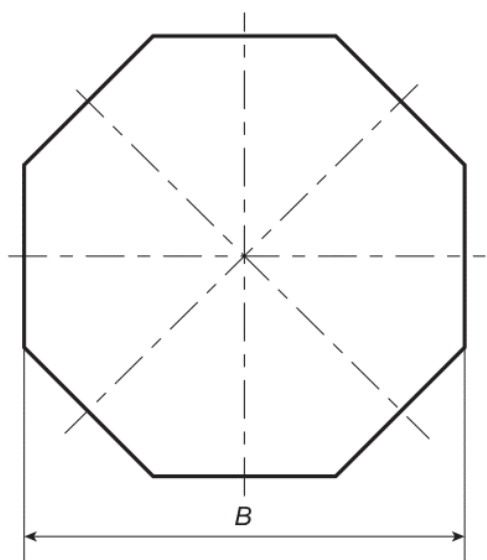
Рисунок Д.3 - Размеры знака 2.5
