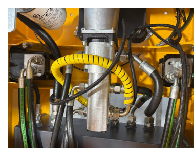
4 гидромотора
