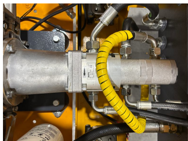
Трехконтурная гидросистема
