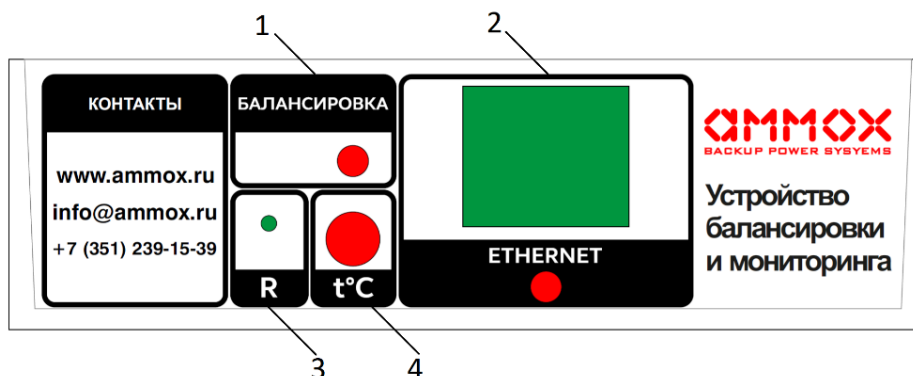
Рисунок 4.1 – лицевая панель модификации BASIC
