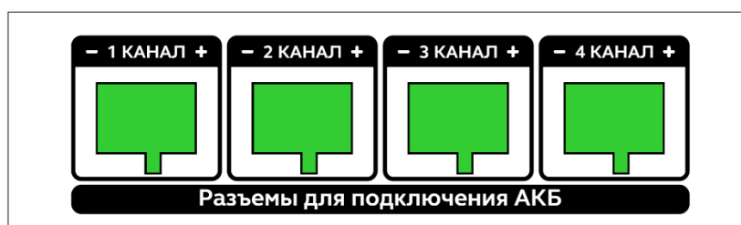
Рисунок 2 – тыльная панель БР-12
