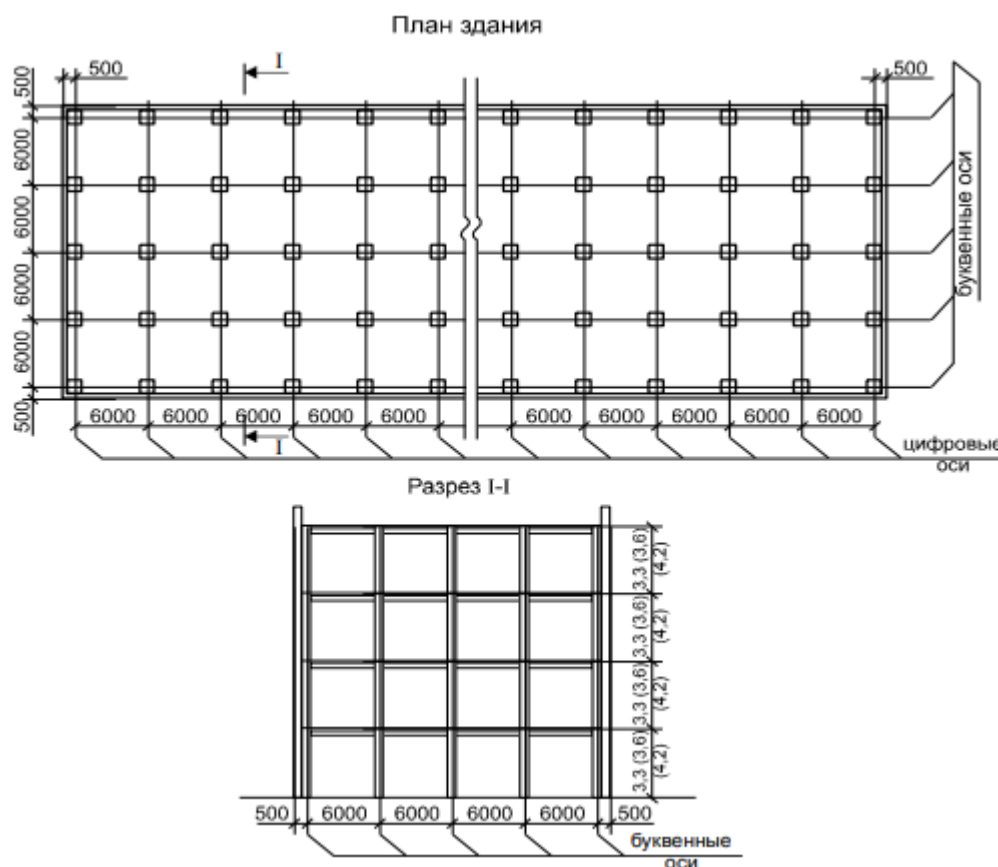
Рисунок 2. Конструктивно-планировочная схема зданий бытового назначения.
