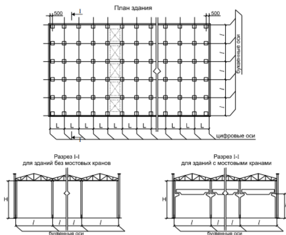
Рисунок 1. Конструктивно-планировочная схема одноэтажного промышленного здания.
