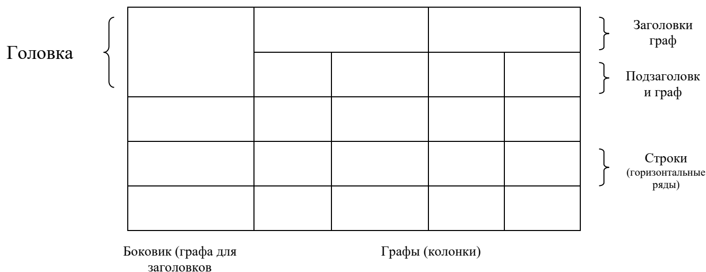
Рисунок 2 – Макет таблицы
