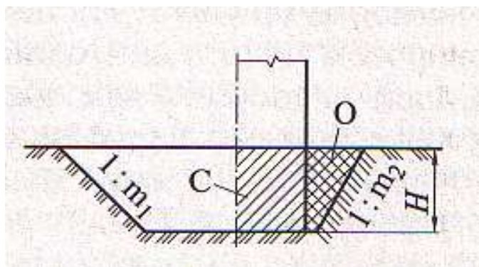
Рисунок 3. Разрез котлована:
