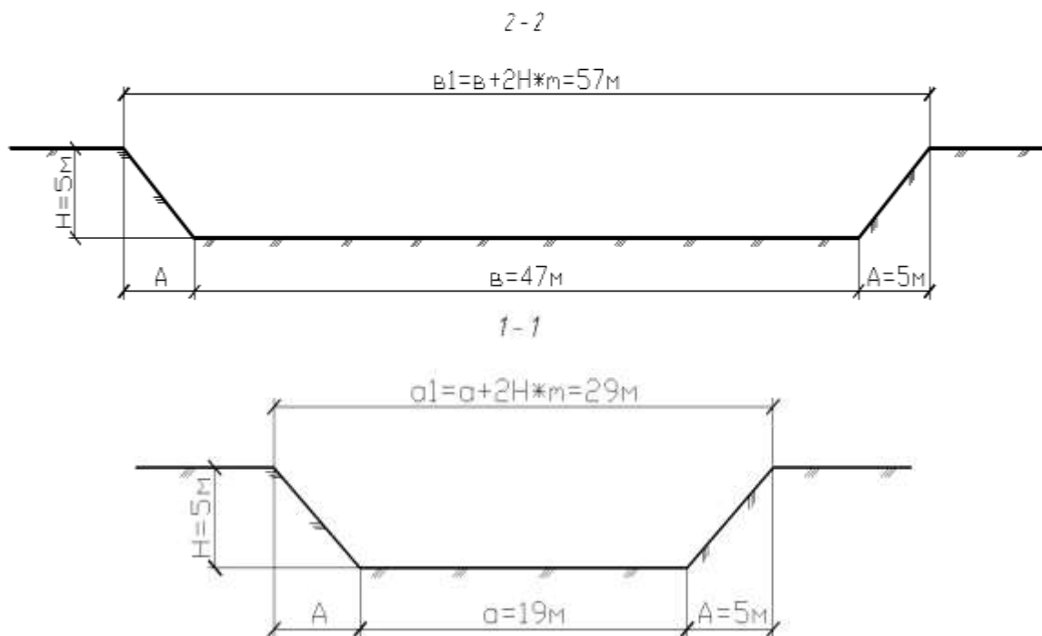
Рисунок 5. План и сечения котлована
