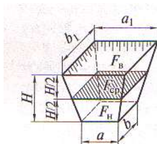
Рисунок 1. Геометрическая схема определения объёма котлована
