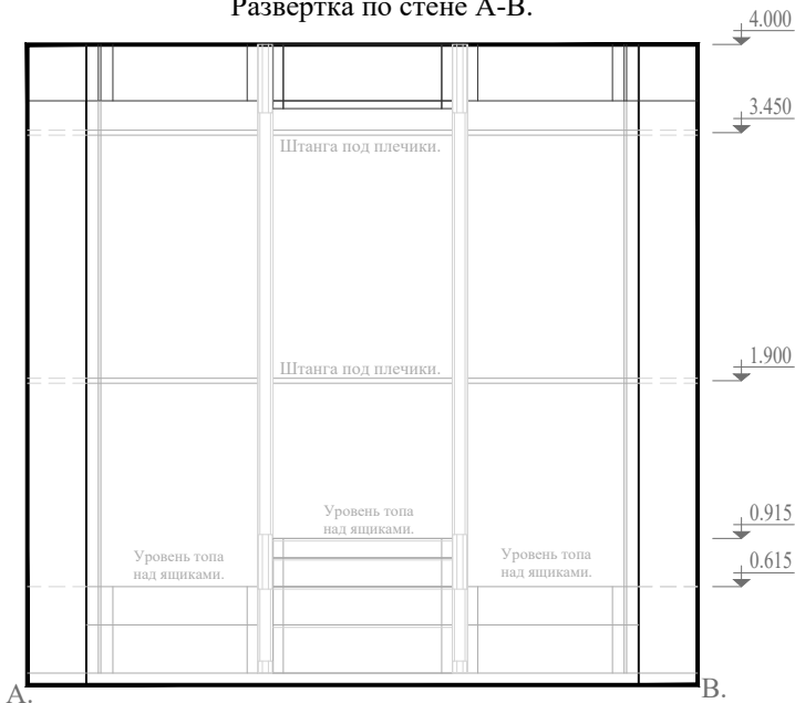
Развертка по стене А-В.
