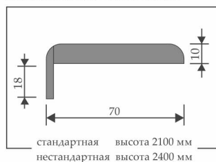
НАЛИЧНИК ПЛОСКИЙ
