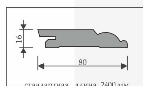
ПЛИНТУС ТИП 3
