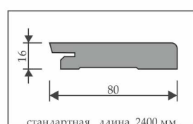
ПЛИНТУС ТИП 1
