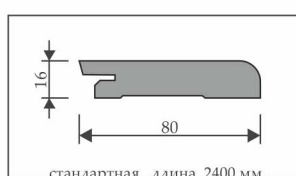
ПЛИНТУС ТИП 2
