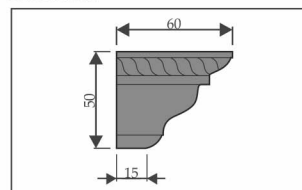
КАРНИЗ
