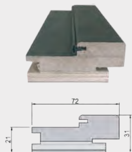
Стойка короба компланарная
