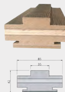
Стойка короба барная
