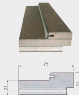
Стойка короба комбинированная
