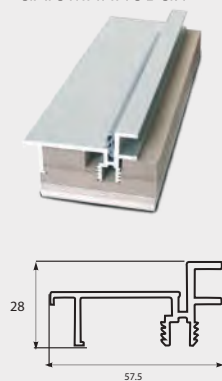
Стойка короба скрытая алюминиевая
