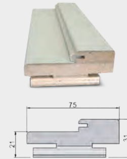
Стойка короба телескопическая
