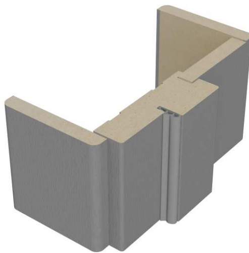
Стандартный погонаж с уплотнителем
