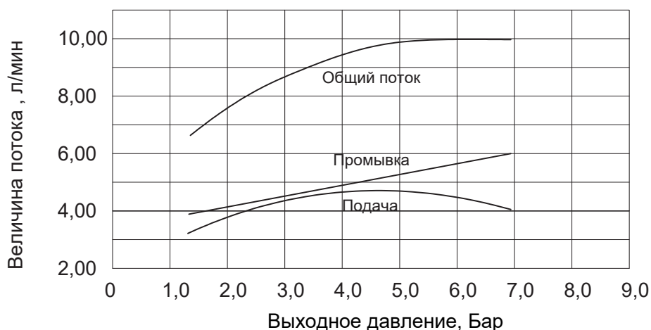
Инжектор 3С 1700/1710
