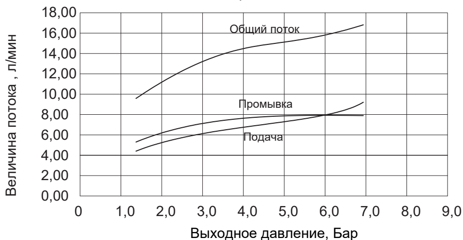
Инжектор 4С 1700/1710
