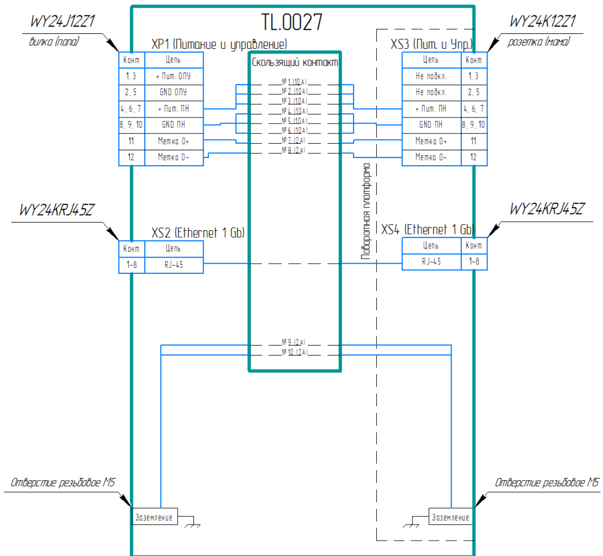
Рисунок 3-б – Схематичное изображение цоколёвки разъёмов ОПУ TL.0027
