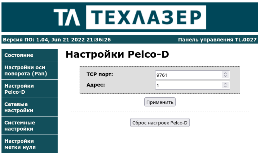
Рисунок 9 – Страница Настроек Pelco-D
