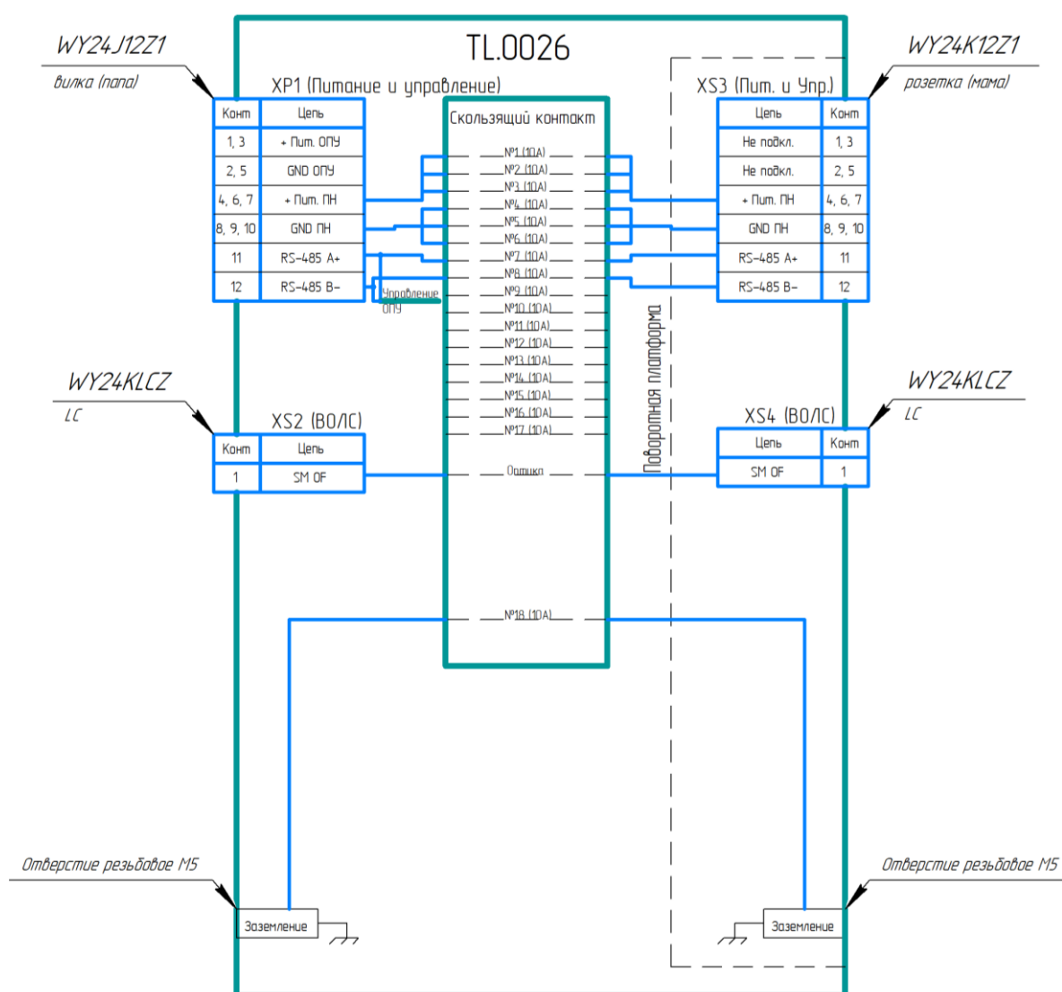
Рисунок 3-а – Схематичное изображение цоколёвки разъёмов ОПУ TL.0026
