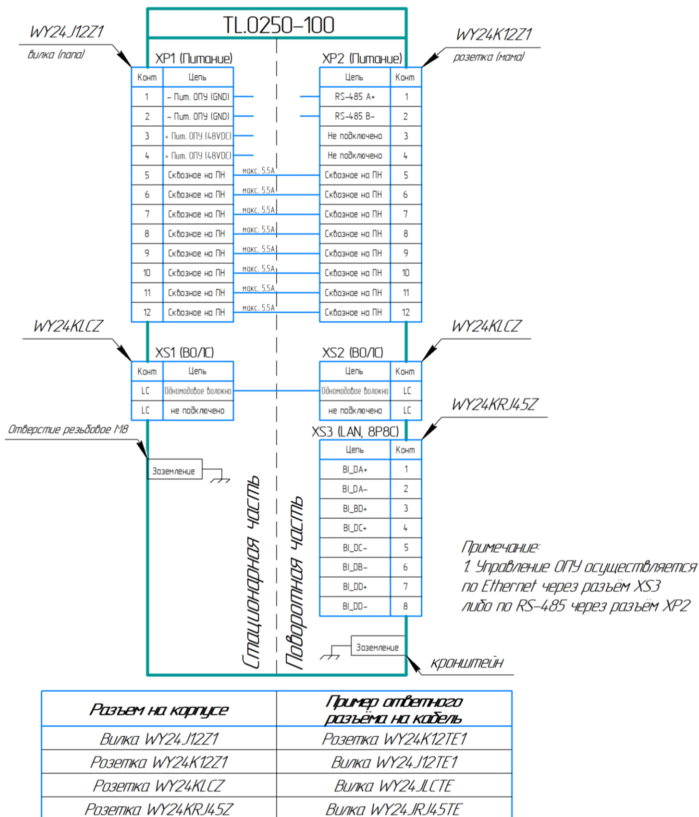
Рисунок В1 – Схема подключений
