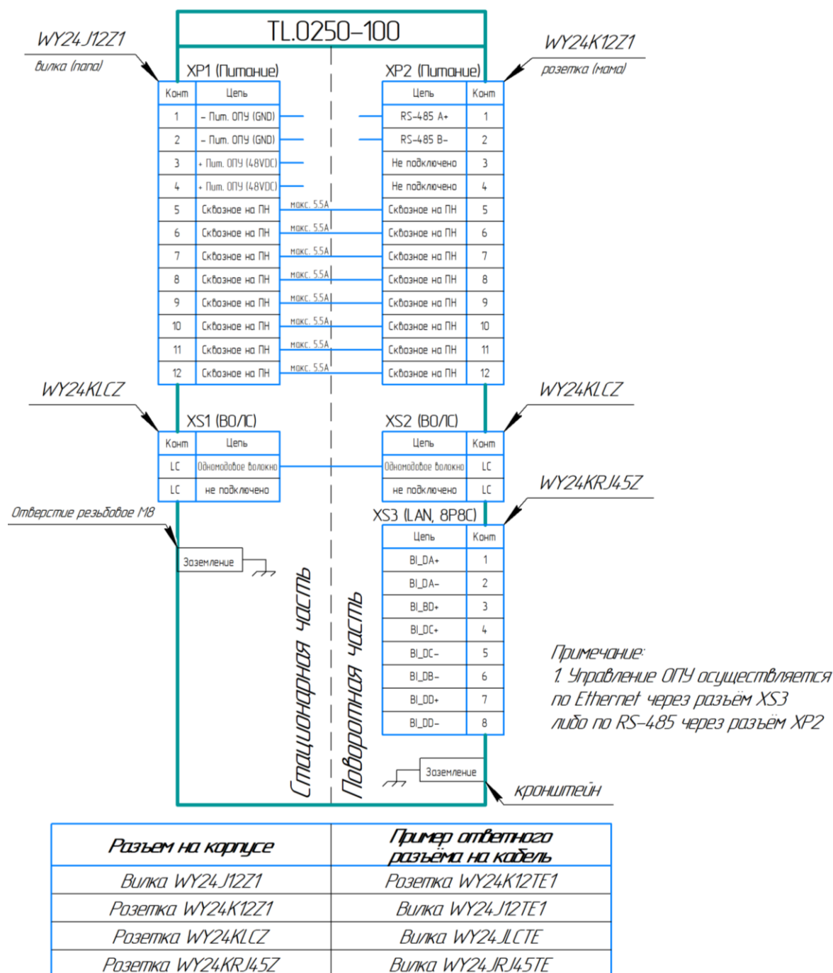
Рисунок В1 – Схема подключений
